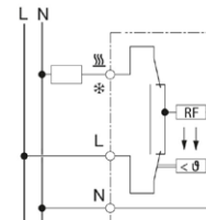
— Schaltbild UTE 1770
