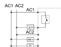
— Schaltbild UTE 2500-24
