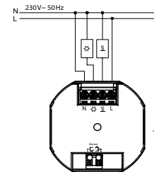
Schaltbild UTE 4800-Rw
