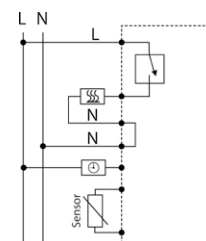
Schaltbild UTE 2800-L
