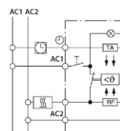
— Schaltbild UTE 1012
