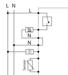
Schaltbild UTE 2800-F
