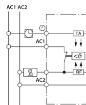
— Schaltbild UTE 1002
