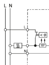
— Schaltbild UTE 1003
