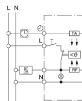
— Schaltbild UTE 1015
